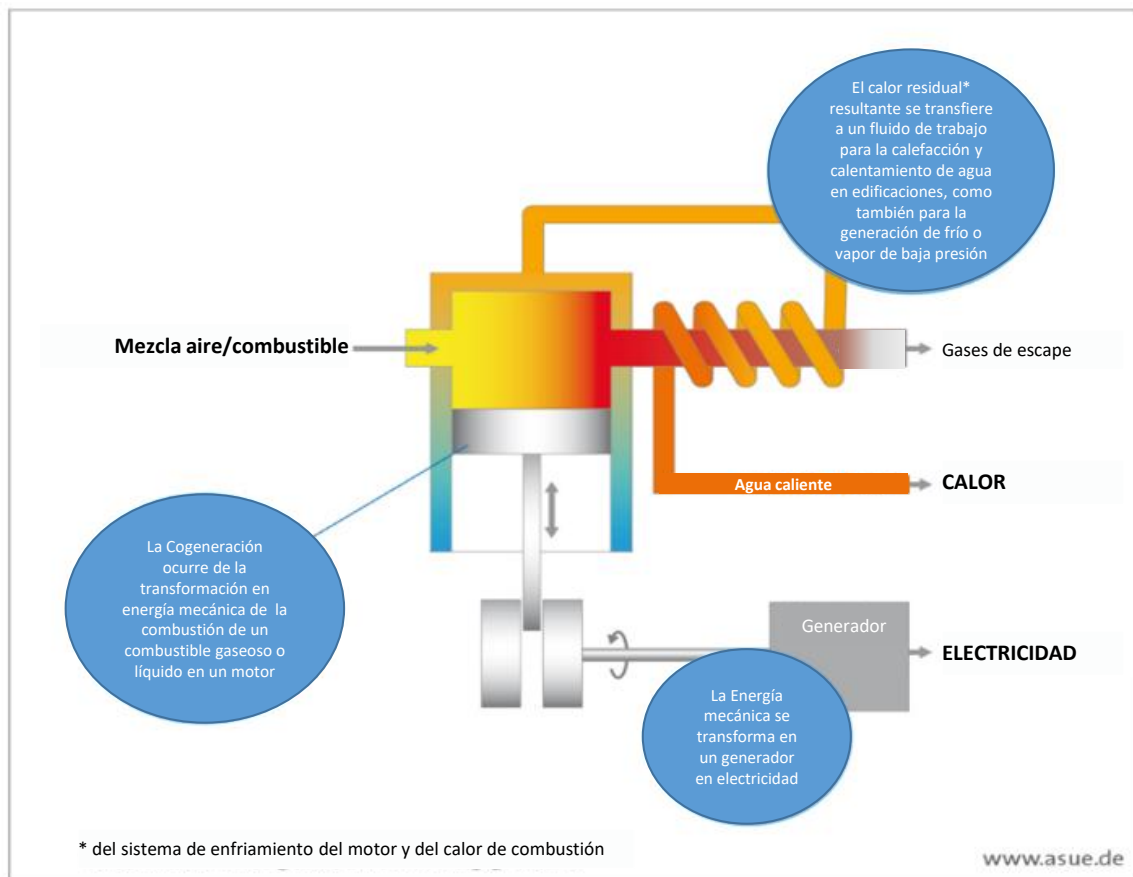
Figura 1 Esquema de motor a combustión de hidrógeno
